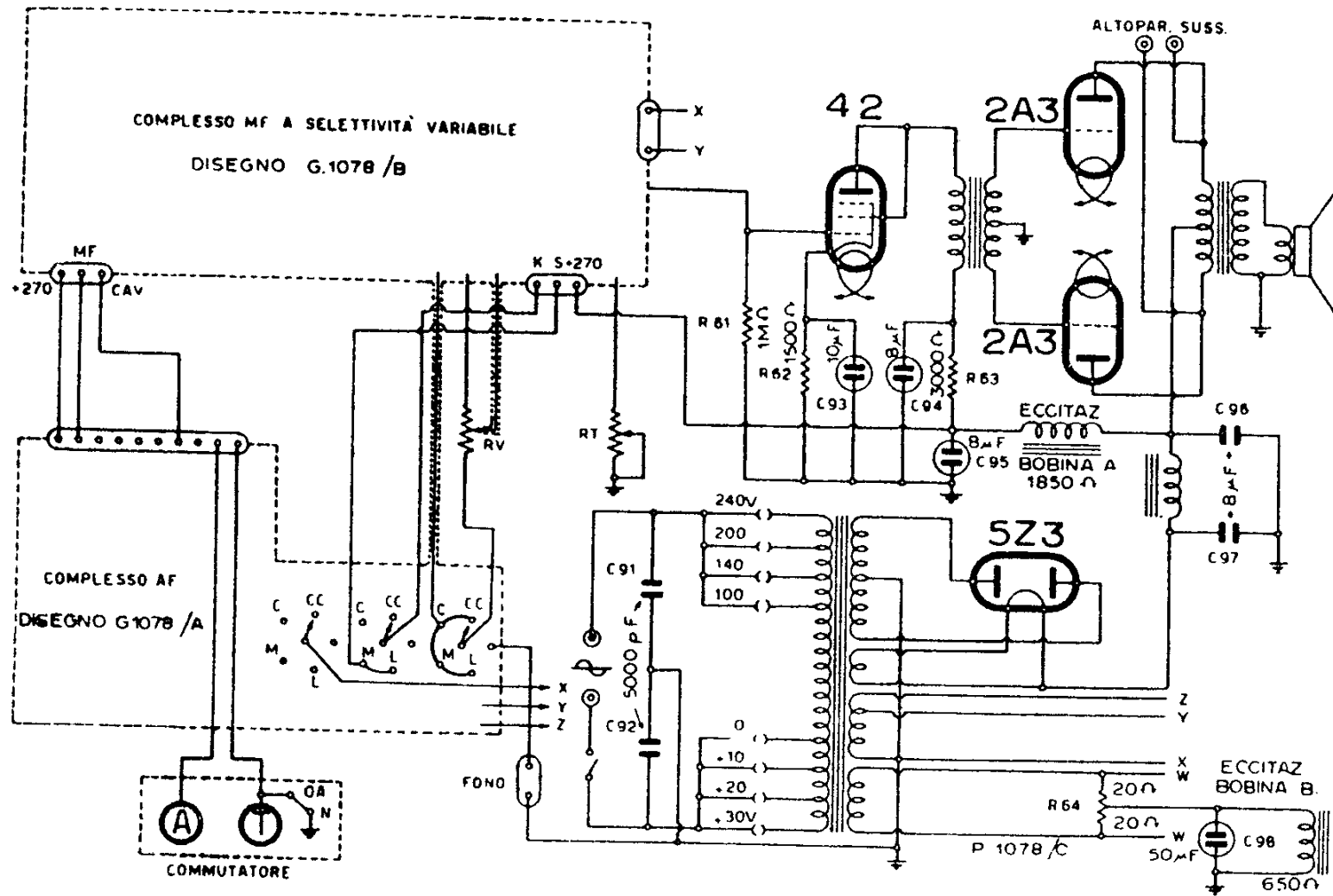
F.I.M.I. - MOD. PHONOLA « 880 » - PARTE BF
